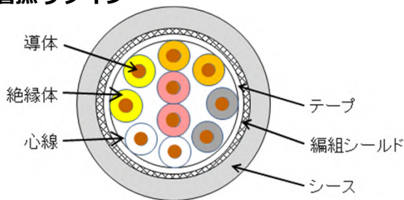
断面図(例) 10心
