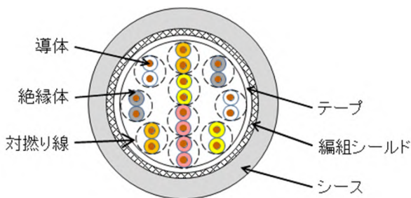
断面図(例) 10対
